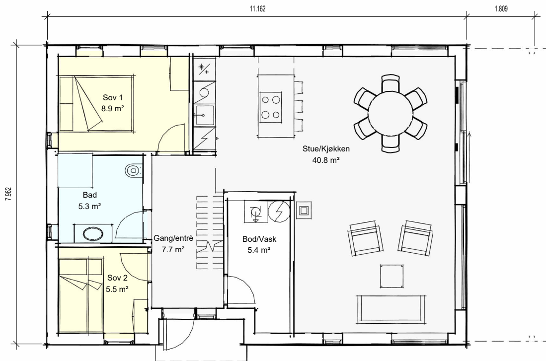
Hovedplan
